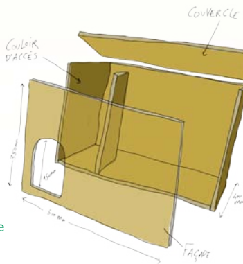
Plan d'un nichoir à Chouette effraie
